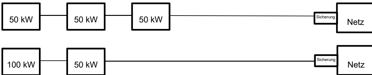
Abbildung 3: Mögliche Kombination in einem 150kW Tauro System
