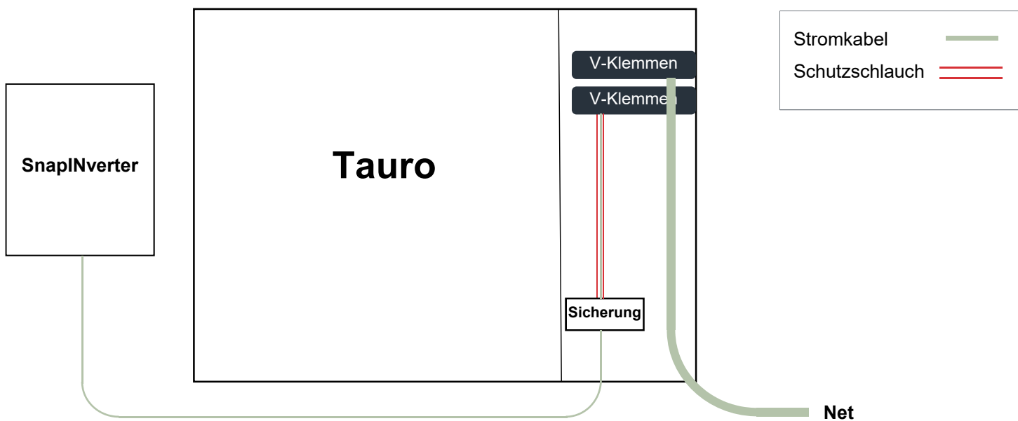
Abbildung 5: Kabelinstallation von SnapINverter Symo 20 und Tauro ECO-100-D
