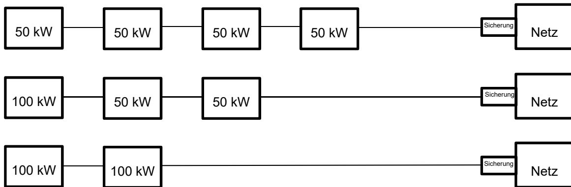
Abbildung 2: Mögliche Kombination in einem 200kW Tauro System
