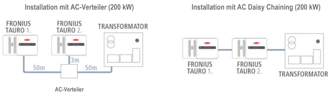
Abbildung 1: Vergleich von Systemdesign 1 mit AC-Verteiler und Systemdesign 2 mit AC Daisy Chaining Option
